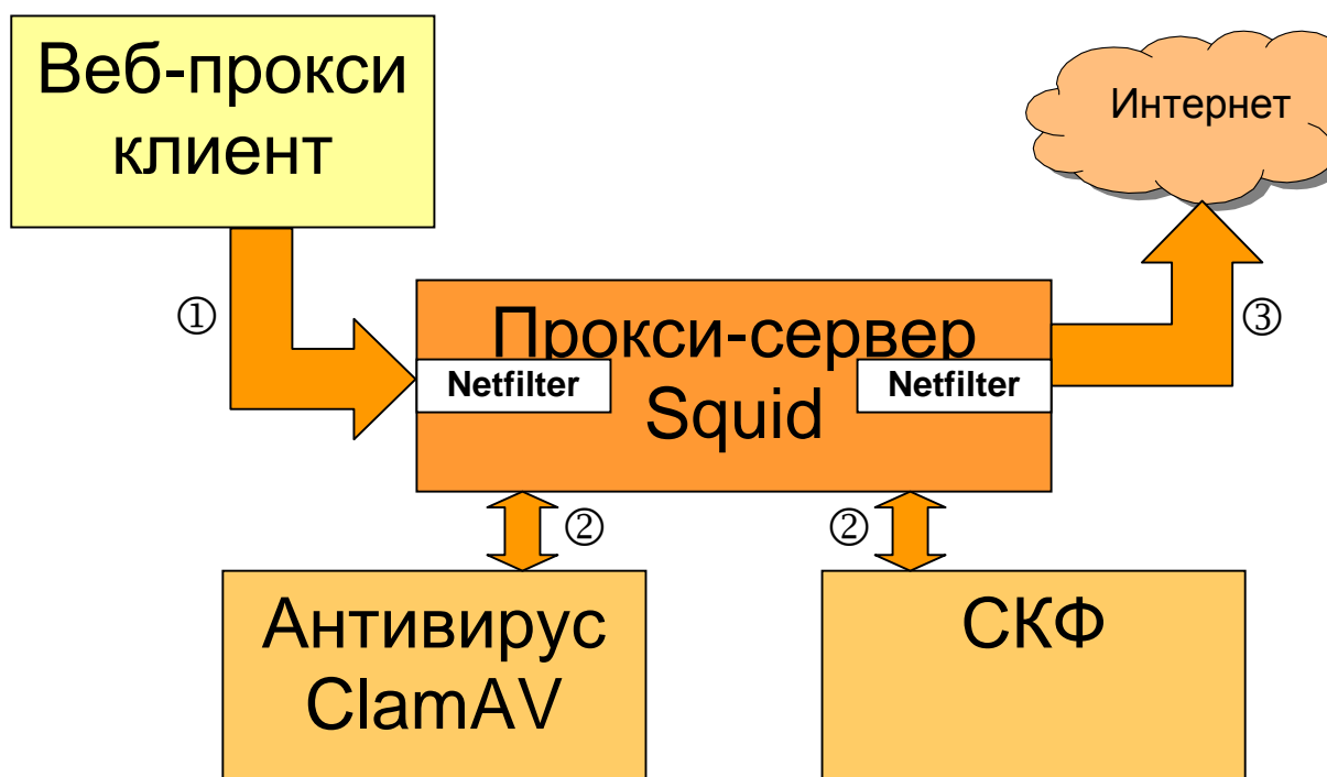
Рис. 3. Схема обработки исходящих запросов из сети образовательного учреждения
